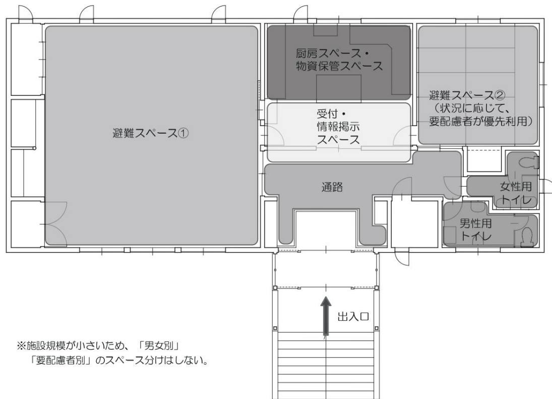
(1) 避難所機能ゾーニング図 [1階]
