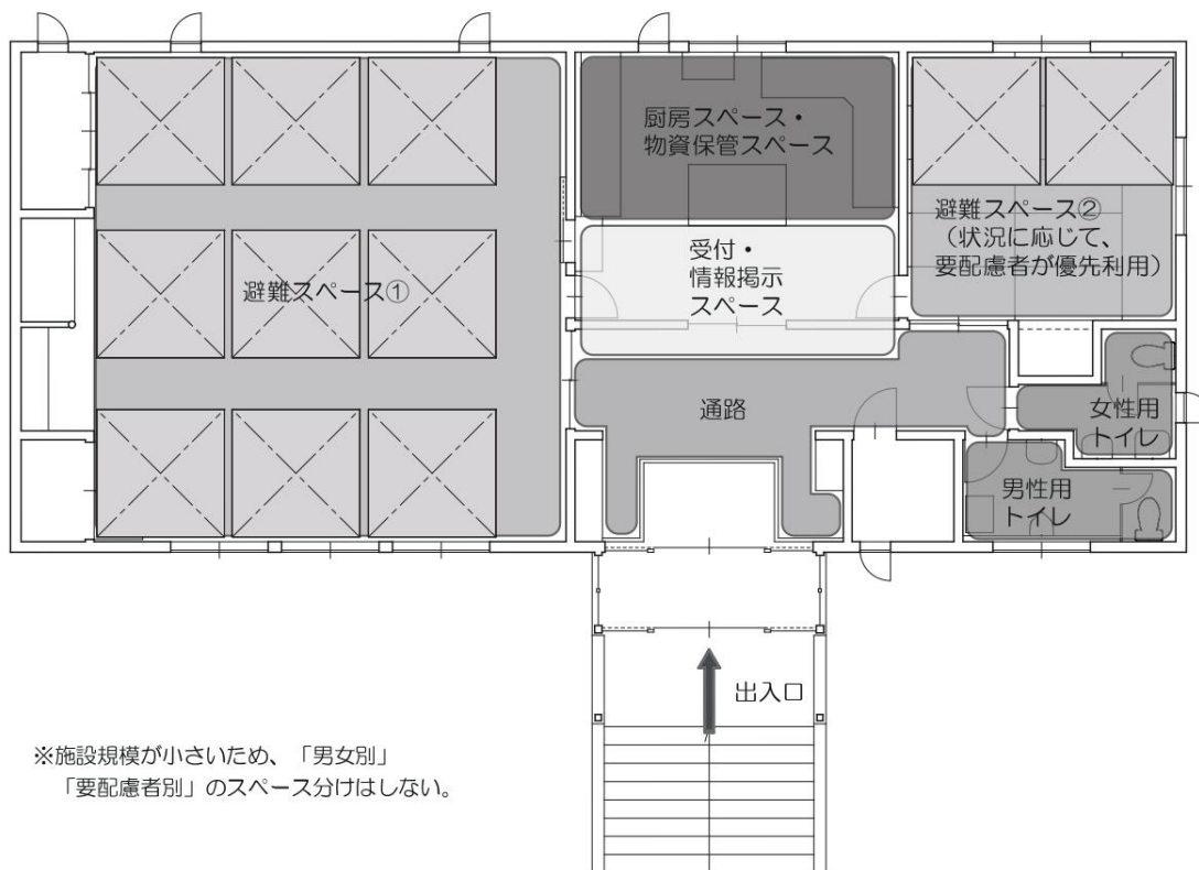
(1) 避難スペースレイアウト図 [1階]
