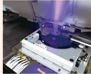
EUV露光装置 提供:ASML
